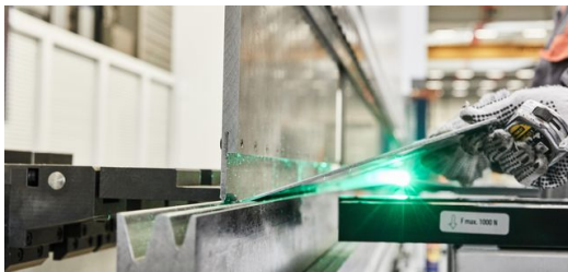
Das Hinteranschlagsystem der neuen TRUMPF EHT VarioPress 500 ist mit Biegehilfen und einer Hochhalteinrichtung gekoppelt, die CNC-gesteuert zum Einsatz kommen. Bild: Florian Bilger
